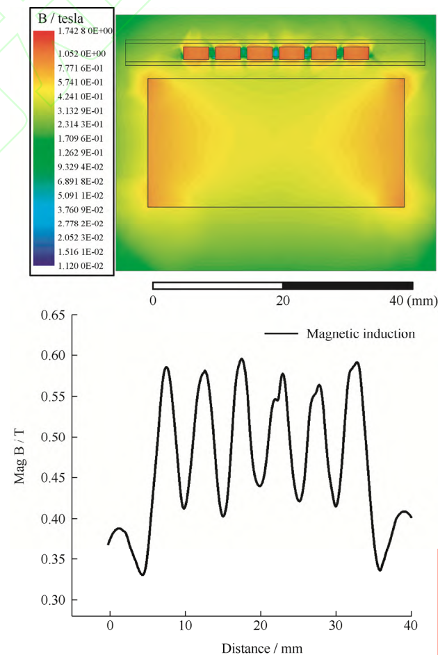
图 2 磁感应强度仿真云图和曲线图
