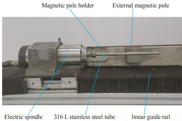
图3 磁粒研磨加工 316L 不锈钢细长管实物图
