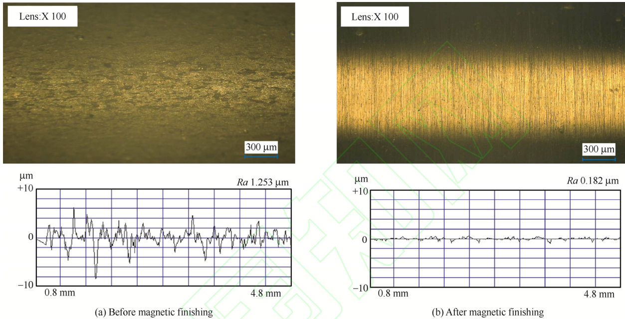
图 10 磁粒研磨 316L 不锈钢细长管前后微观形貌及表面粗糙度
