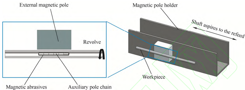
图 1 磁粒研磨加工 316L 细长管原理
