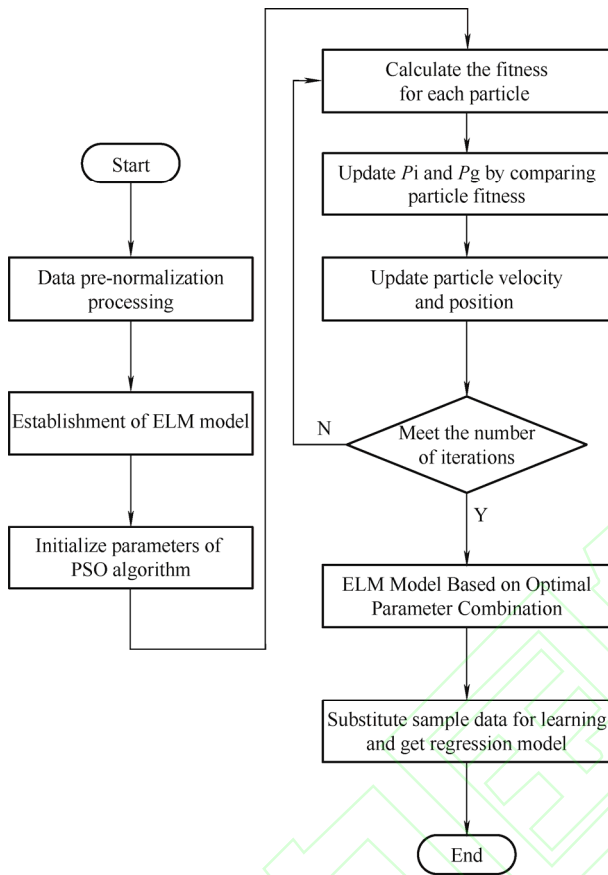
图 4 PSO-ELM 流程图
