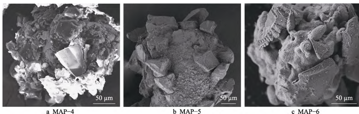
图7 不同温度下磁性磨粒的SEM图
